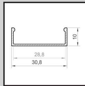
Řez LED profilu (jednotky: mm)
